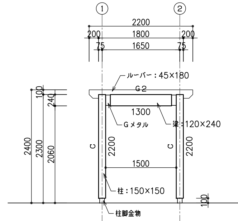
A通り軸組図 1:50
