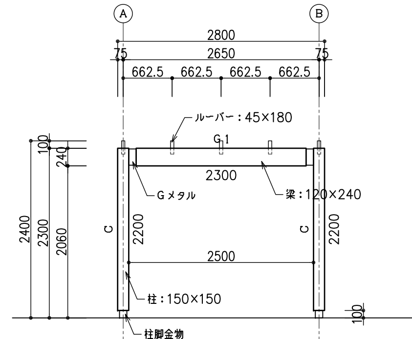
1通り軸組図 1:50
