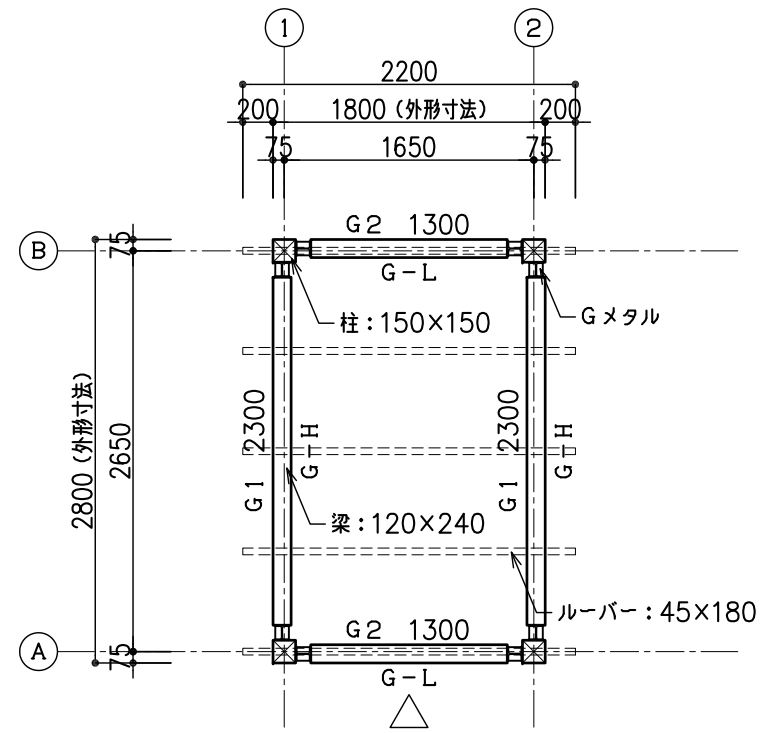
梁伏図 1:50
